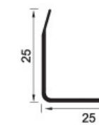
KST-Z25A Weight: 0.13kg/m
